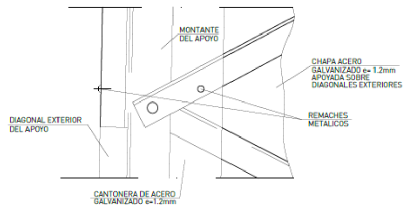
DETALLE SECCION B-B FIJACION ANTIESCALO ESCALA 1:5
