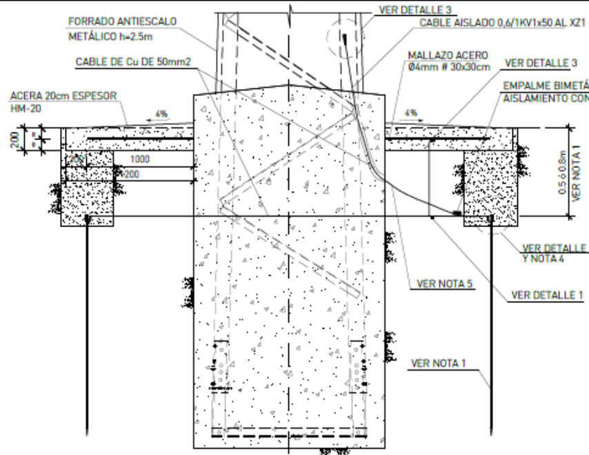
DETALLE 1 SIN ESCALA
