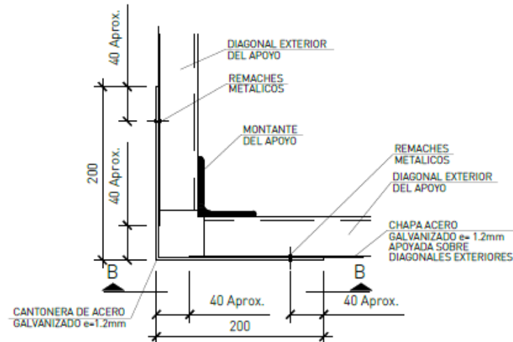
DETALLE PLANTA FIJACION ANTIESCALO ESCALA 1:5
