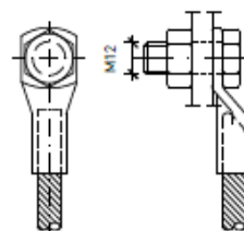
DETALLE 3 SIN ESCALA
